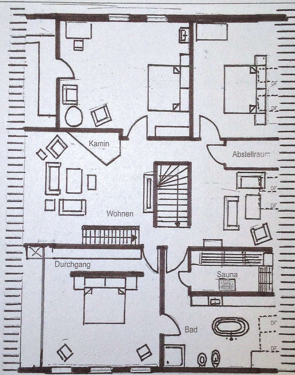
Hauptgebäude Obergeschoss
